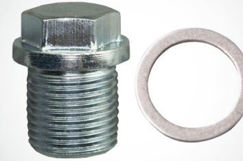
670-P6112127X M18x1,5x18 8212127A 18x24x1,5
